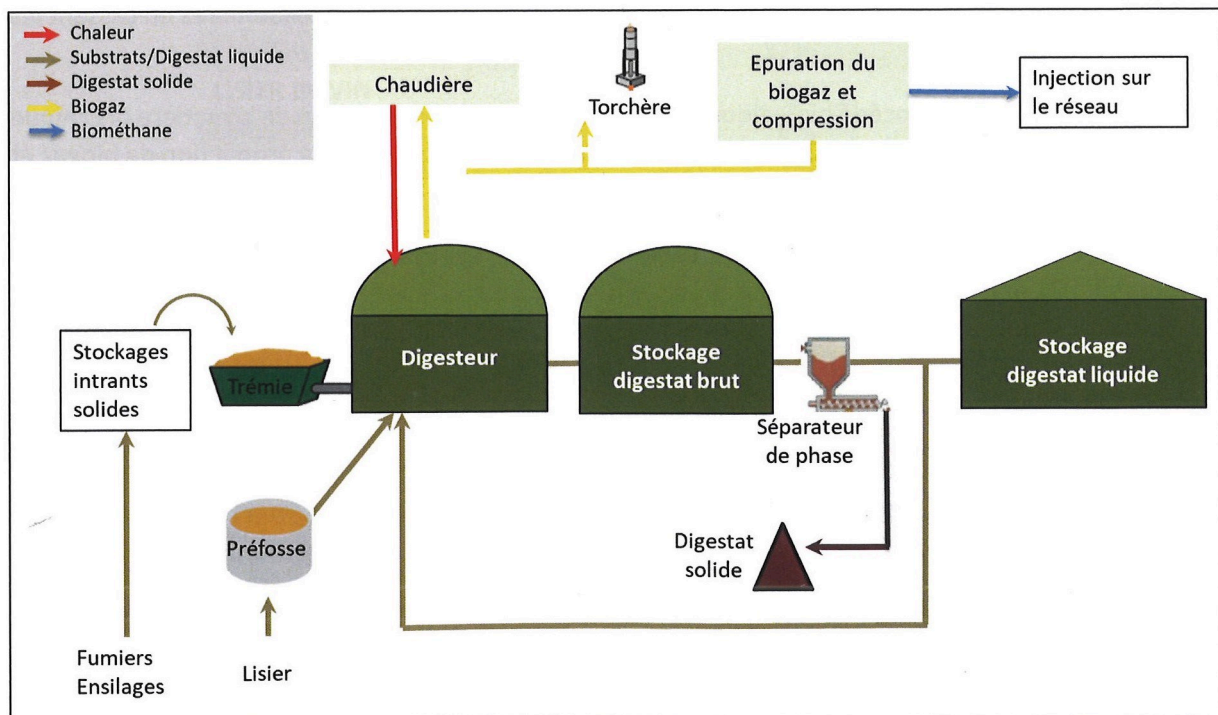
SCHEMA DE PRINCIPE DE L'INSTALLATION DE METHANISATION
